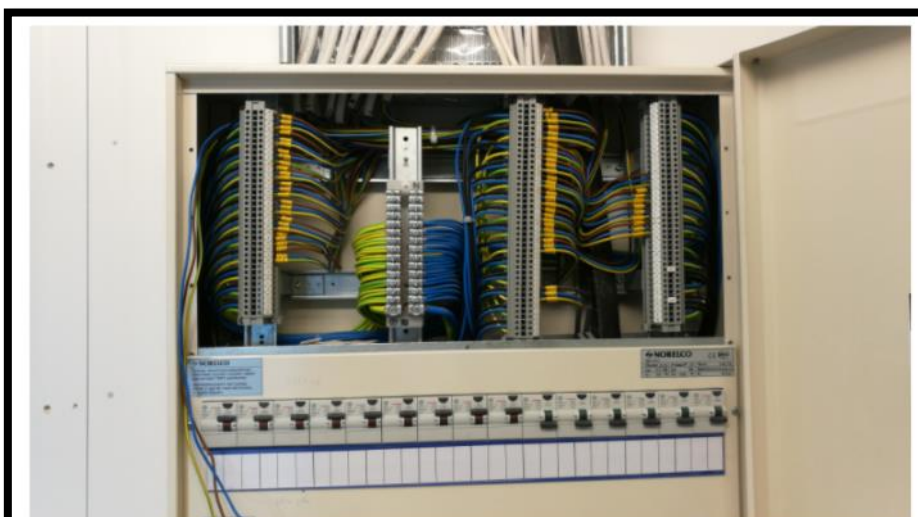
Fra et tidligere eltilsyn i Trondheim: Splitternytt anlegg med 1-polte sikringer uten brudd på N-leder. (Foto: Elektroarbeidernes Fagforening Trøndelag)
